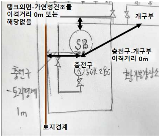
[ 그림 2 ] 소형저장탱크 이격거리 표시 적정 예시
