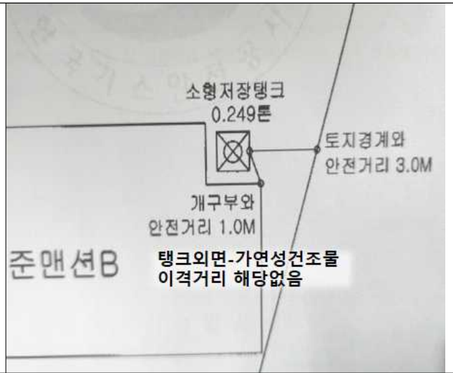
[ 그림 2 ] 소형저장탱크 이격거리 표시 적정 예시
